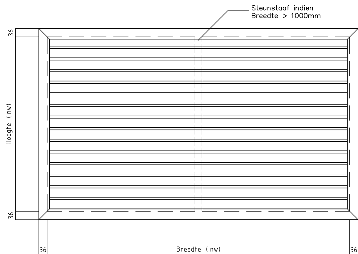
Vooraanzicht
